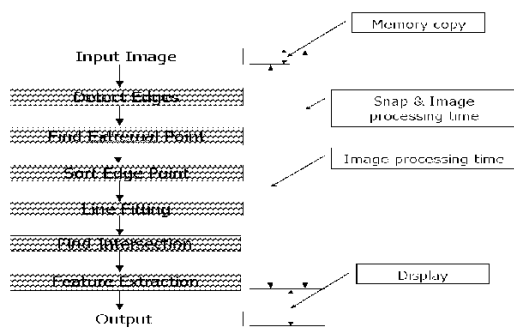
그림 2. 검사 알고리즘
