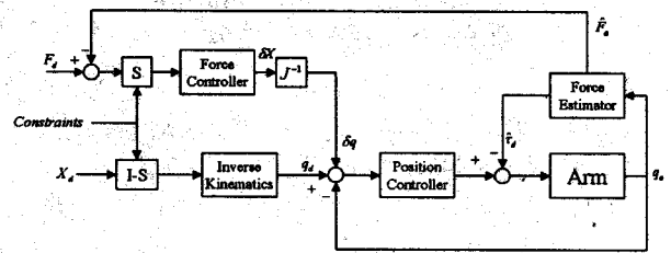
그림 5 힘 추정기를 이용한 하이브리드 위치/힘 제어에 관한 블록도
