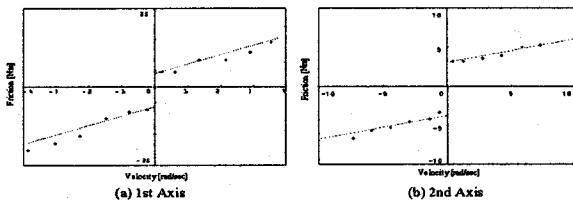
그림 11 점성력 모델 Fig. 11 Friction Model
