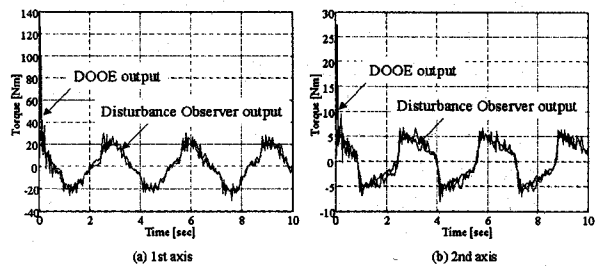
그림 13 DOOE의 출력과 외란 관측기의 출력 Fig. 13 The output of DOOE and the output of disturbance observer
