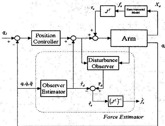
그림 4 힘 추정기에 대한 블록도 Fig. 4 The Block Diagram of Force Estimator
