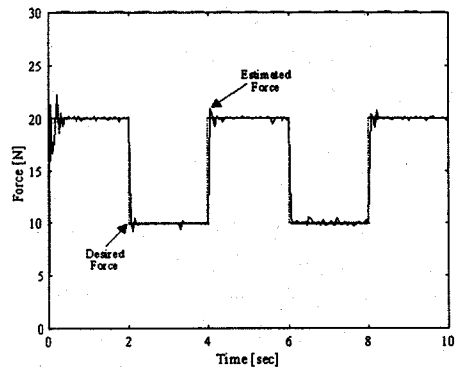
그림 14 제안된 힘 추정기에 의한 힘 응답 Fig. 14 The force response using the proposed force estimator
