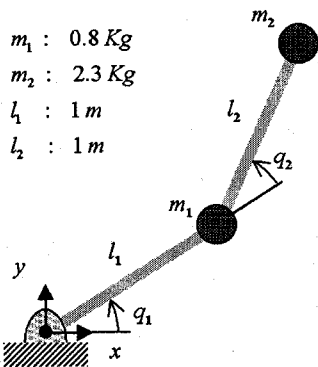
그림 6 2자유도 로봇 매니플레이터 Fig. 6 A two DOF planar type robot manipulator
