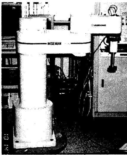
그림 1 2자유도 수평다관절형 직접구동형 로봇 Fig. 1 Two DOF SCARA type direct-drive arm
