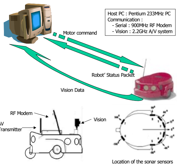
그림 6. 제어 시스템과 모바일 로봇 Fig. 6. Control System and Mobile Robot
