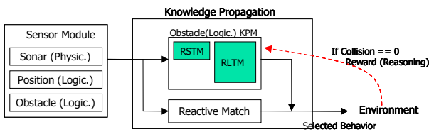
그림 3. 지식 전파 모듈 Fig. 3. Knowledge Propagation Module
