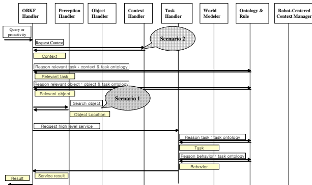
그림 8 Sequence Diagram
